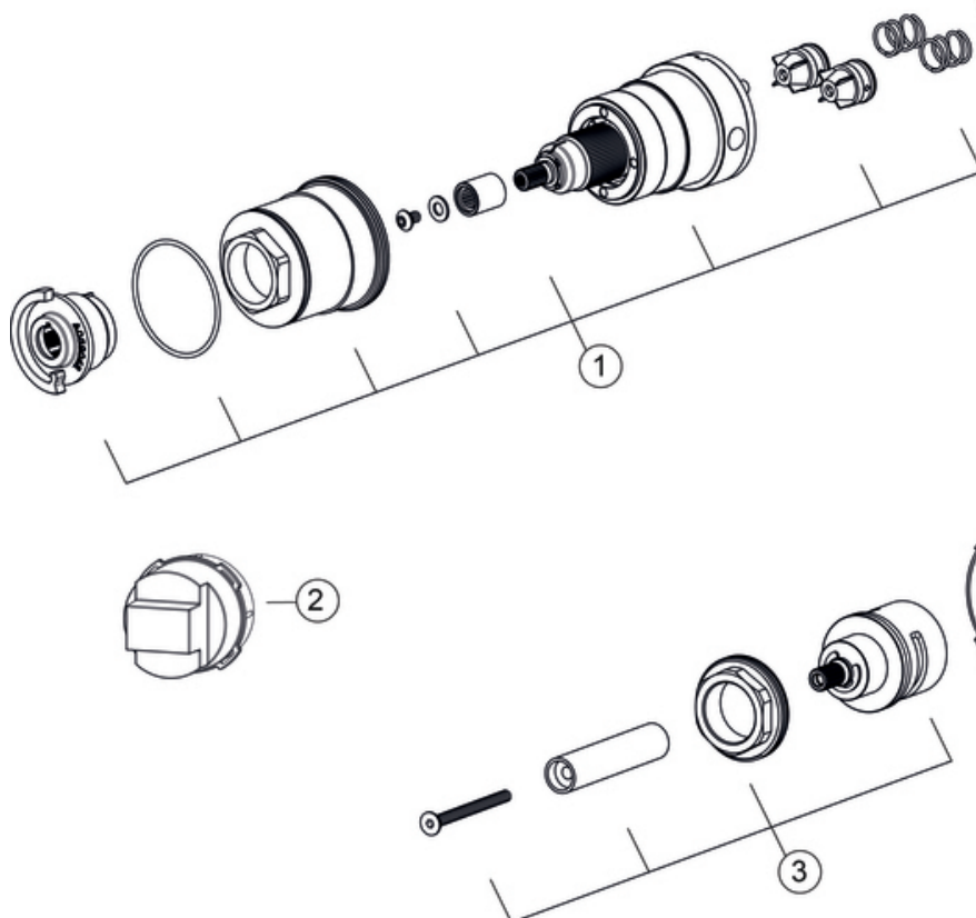
UMSTELLER-MODUL
