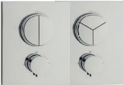
11.803050.2.01 / 11.803055.2.01 Thermostatmischer PUSH Unterputz square Farbset Wandmontage für 2 oder 3 Verbraucher mit PUSH-Buttons Heißwassersperre 38° C | Blende 160 x 130 mm concealed thermostat mixer with push buttons final assembly set for 2 or 3 consumer safety stop at 38° C | cover 160 x 130 mm
