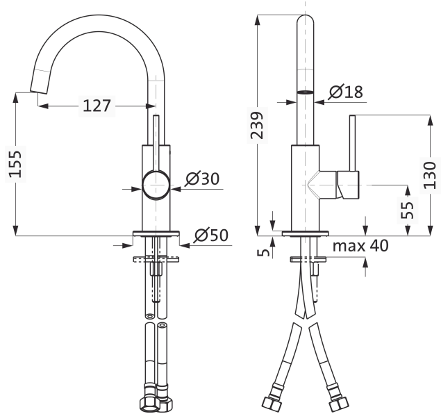
Lochbohrung 35mm
